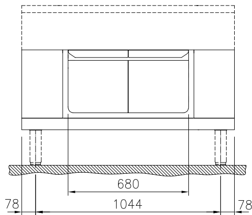
Front aanzicht
